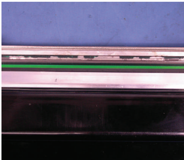
Imágenes mostrando daños en el cabezal de impresión, que se pueden producir usando cintas no Zebra
